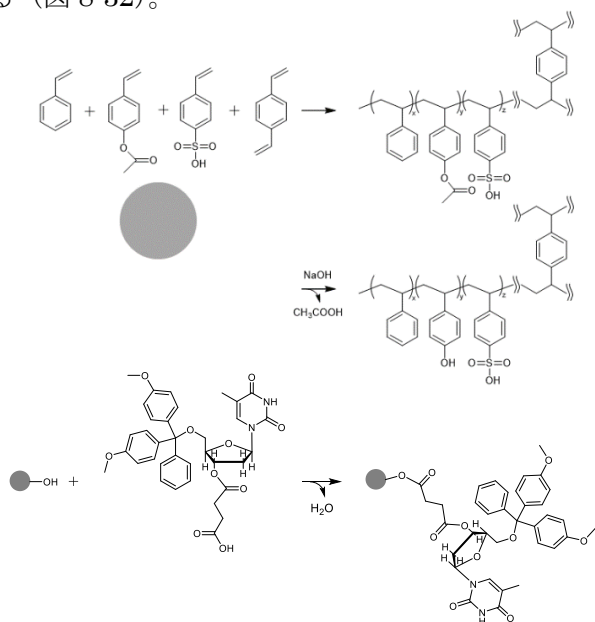
図 8-32 懸濁共重合で得られるマイクロファイアに 1 個目の単量体を縮合する反応。
