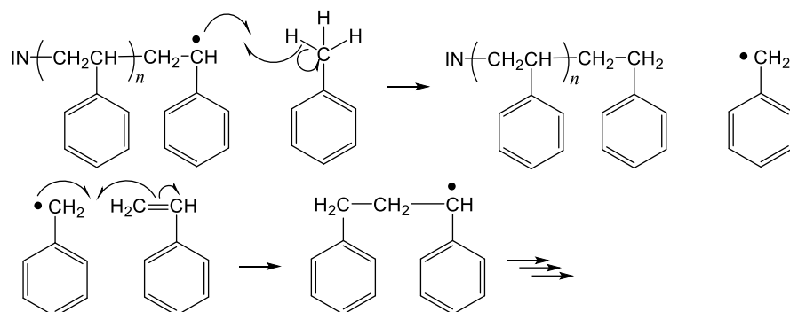
図 8-16 スチレンのラジカル付加重合の際に起こる連鎖移動反応 (溶媒のトルエン C_6H_5-CH_3 がラジカルとなり新たな開始剤となるケース)。高分子の分子量が小さくなり、その分布もばらついてしまう要因となる。
