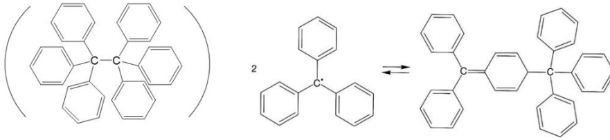
図 8-3 トリチルラジカルの 2 量体の可逆反応。
