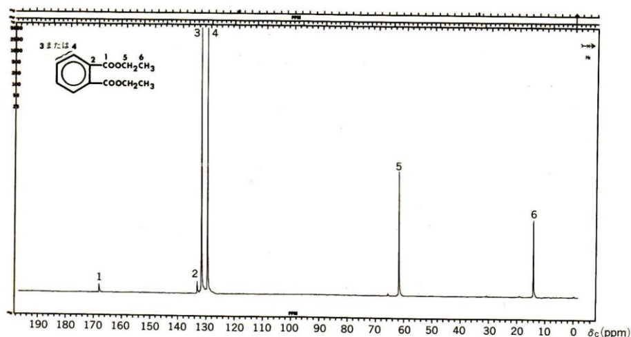
図 5・1(b) 広帯域デカップラーによってプロトンを完全にデカップルしたフタル酸ジエチルの ^{13}\text{C} NMR スペクトル（溶媒 \text{CDCl}_3 , 25.2 MHz）
