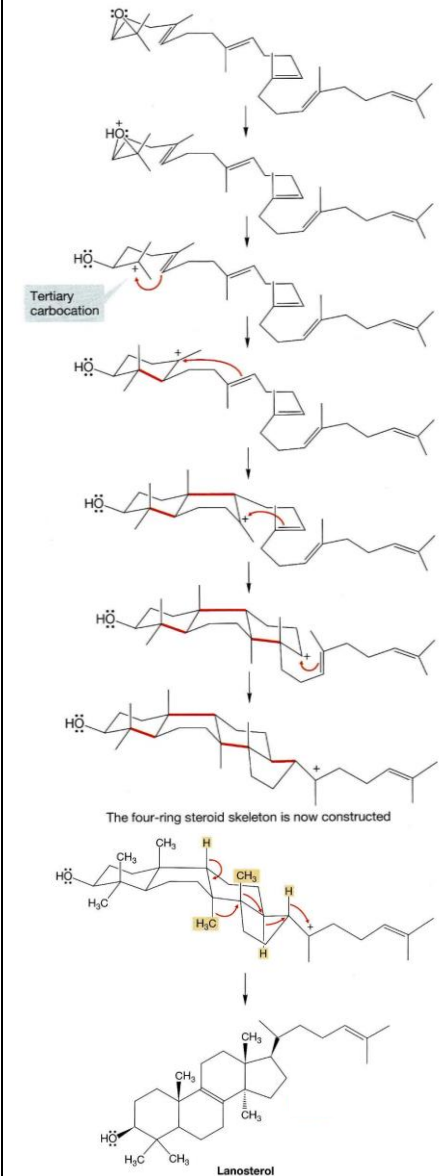
図 4-39 酵素のない環境でカロテノイドやステロイドが生成する連鎖的な反応の経路（オリソンと中谷のモデル）。
