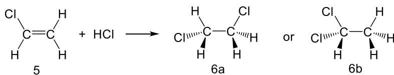
図 4-9 5 と塩化水素との付加反応。
