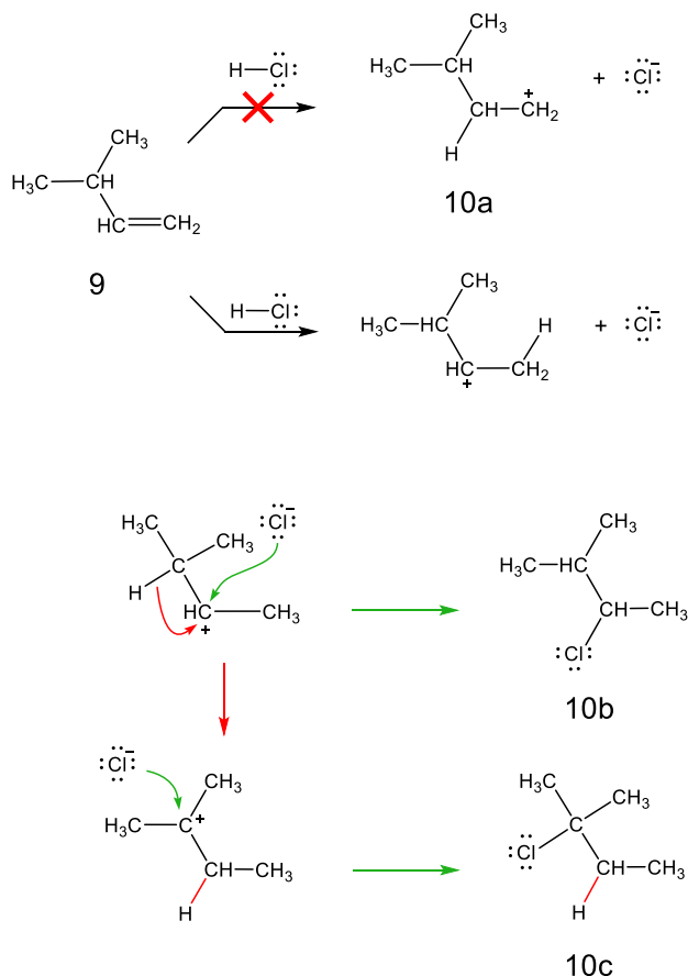
図 4-13 9 と塩化水素との付加反応。
