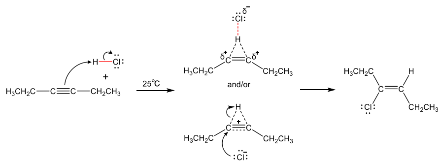
図4-29 3-ヘキシンの塩化水素との付加反応 (1 : 1 の物質質量比で反応した場合)。
