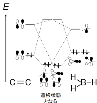
図 4-25 C=C 結合の \pi 電子の分子軌道とボランの分子軌道との遷移状態
