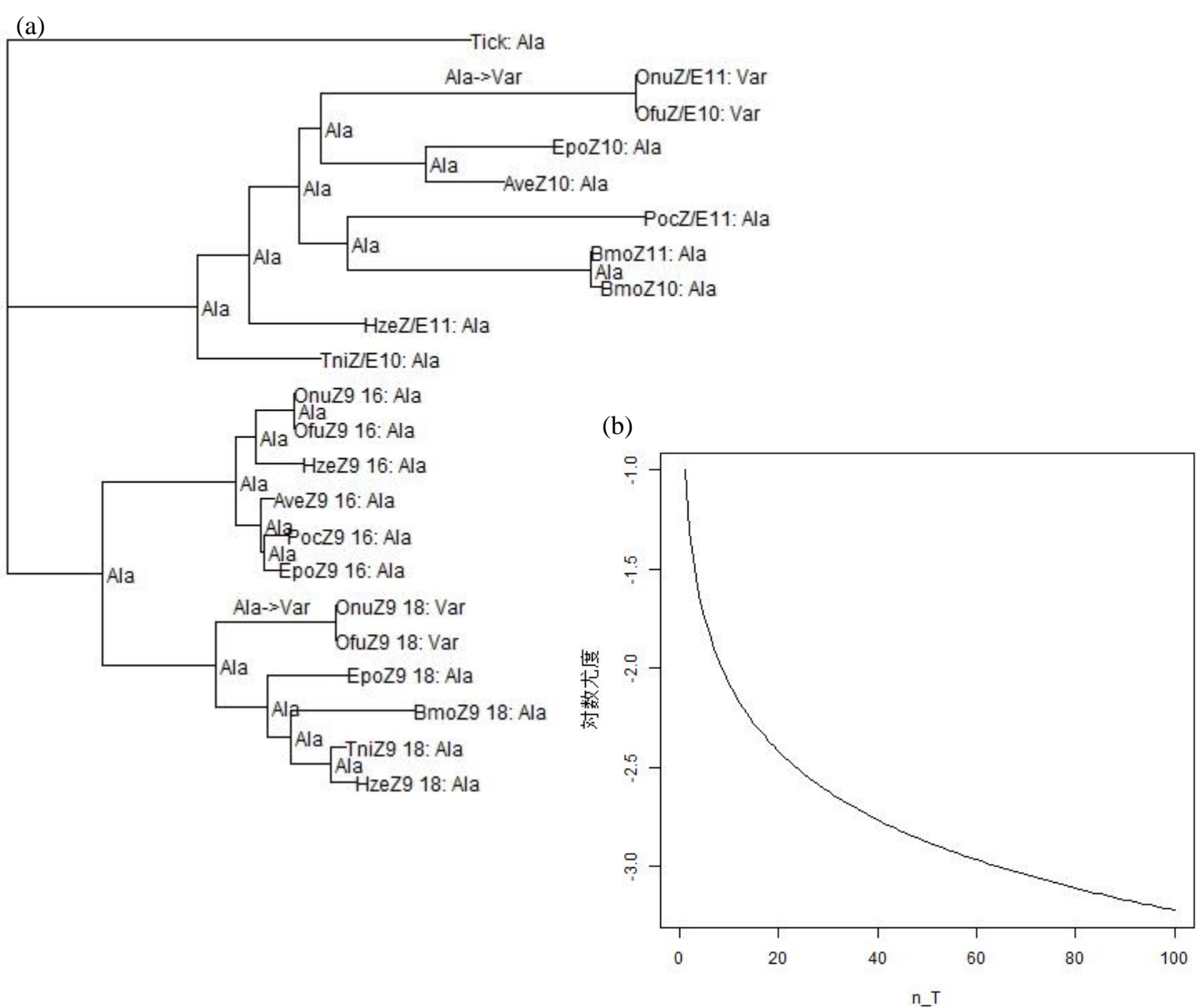
図6.15 最小進化の規準と最尤法
