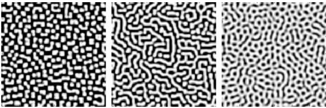
図5.6 反応拡散方程式の実行例 (Wikipedia「チューリングパターン」より) 近藤研究室の反応拡散シミュレータにより、同様のパターンを自在に作成できる。
