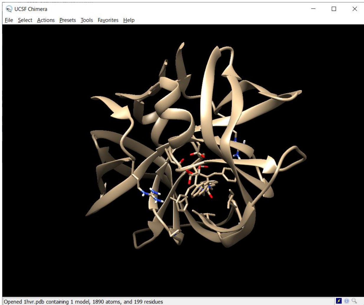
図4.2 UCSF Chimeraで1hrv.pdbを開いた様子
