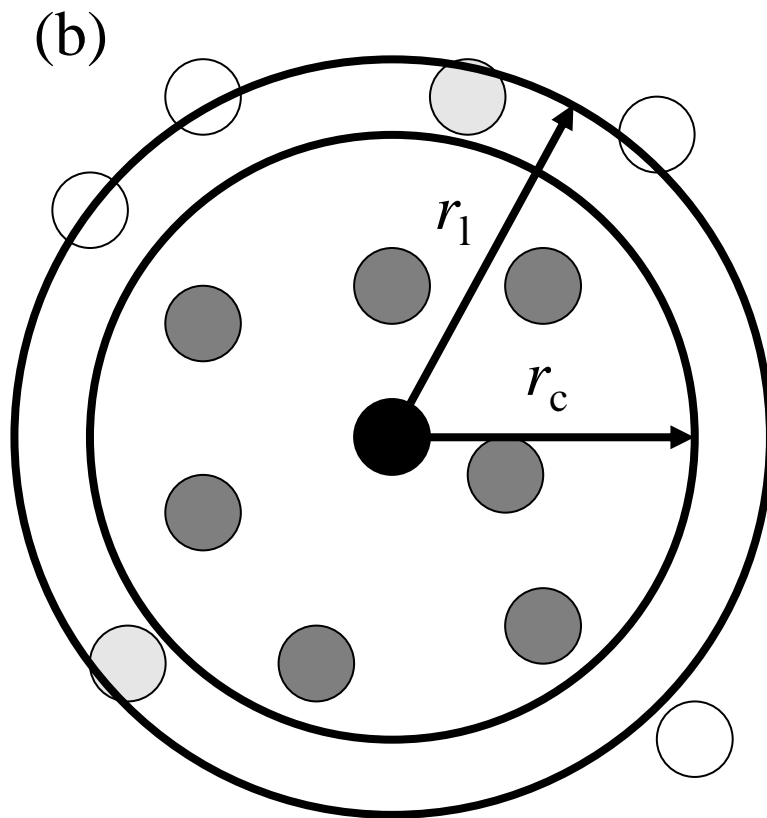
図4.16 (a) カットオフ法 中央の原子（黒色）から距離 r_c 以内にある原子（暗灰色）との相互作用を計算する。(b) ペアリストの作成 中央の原子（黒色）から距離 r_l 以内にある原子（明灰色と暗灰色）とのペアリストを作成し、その中で、距離 r_c 以内にある原子（暗灰色）との相互作用を計算する。
