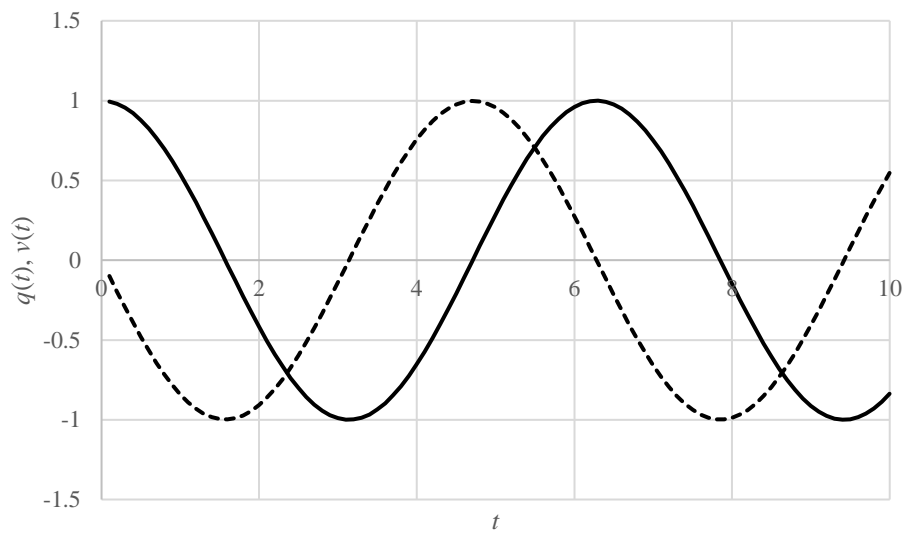
図4.13 \Delta t = 0.1 としたときの調和振動子ののび q （実線）と速度 v （破線）の時間変化
