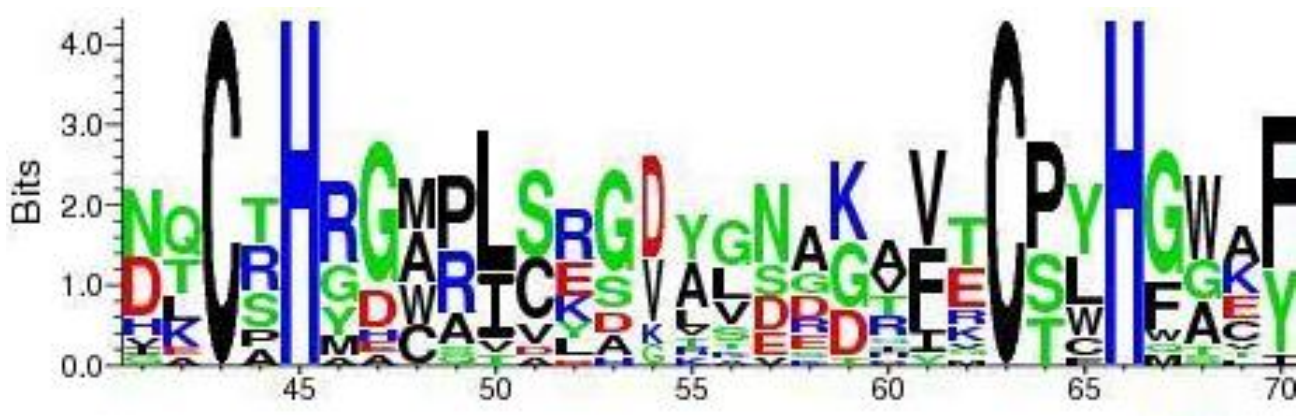
図3.33 Rieske型鉄硫黄クラスター結合部位の一部のシーケンスロゴ
