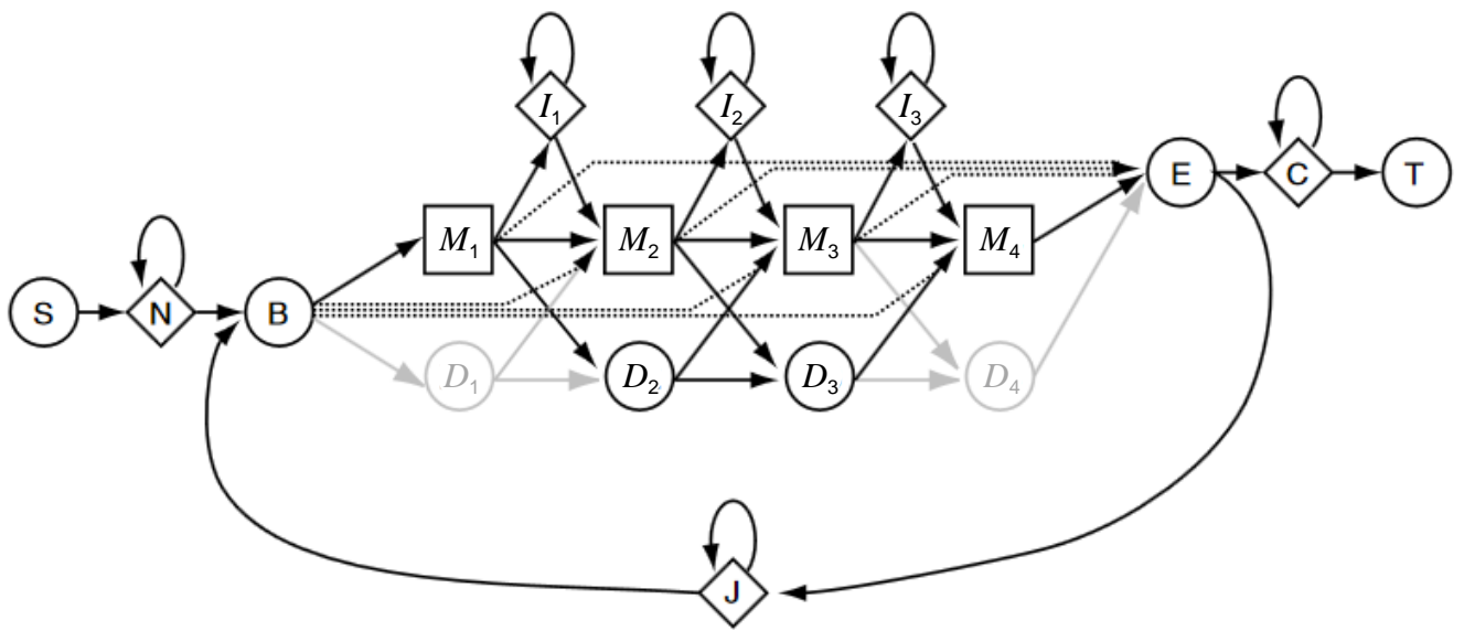
図3.27 HMMERで用いられているプロファイルHMMの一般形 (Eddy SR., 2003を一部改変)
