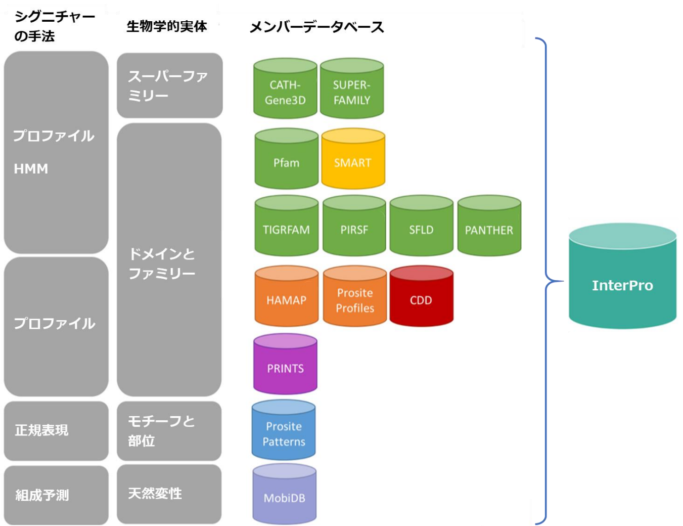
図3.18 InterProの構成
